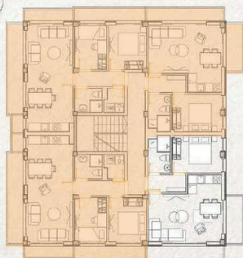
ОСНОВА НА ПОТКРОВЈЕ
